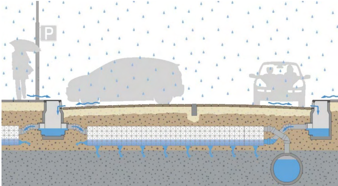
Figuur 11 - Infiltratiekratten
